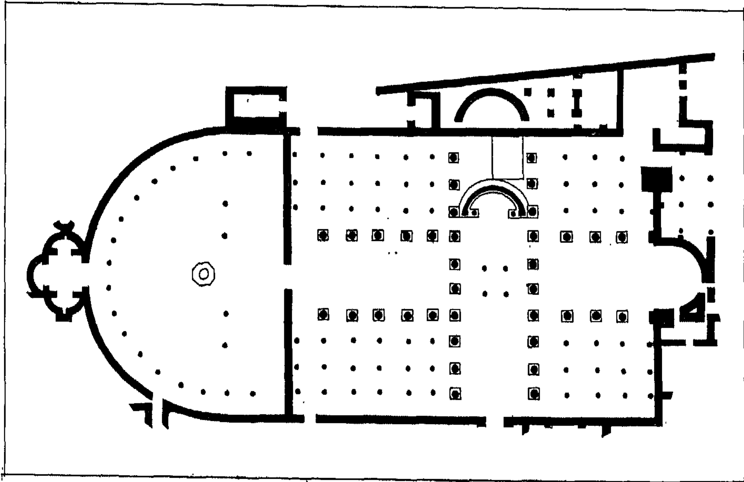
(شكل ٦) رسم تخطيطي لكنيسة داموس الكاريتيه
