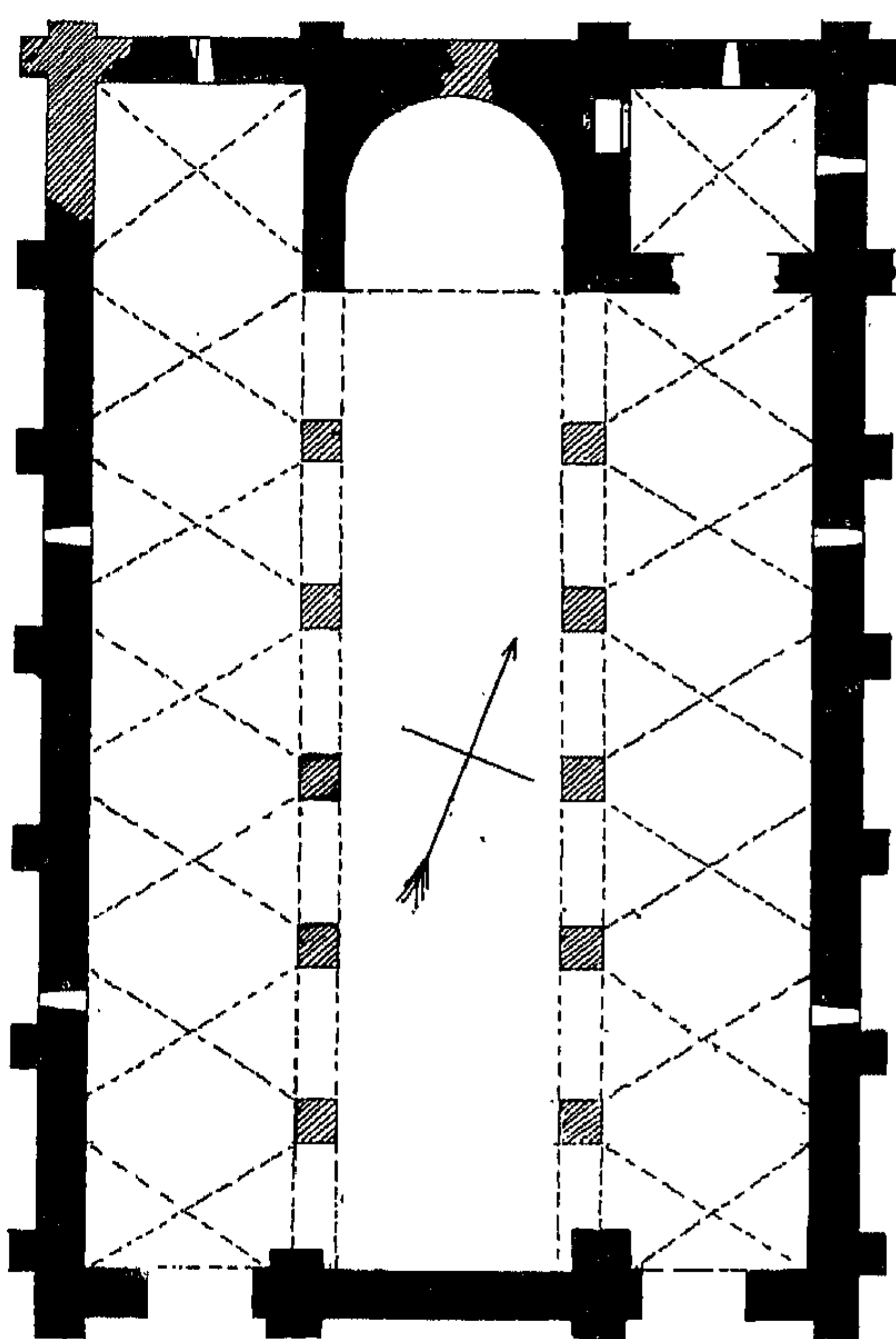
(شكله) رسم تخطيطي لكنيسة قصر المحر
