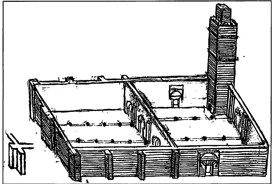
لوحة مجمعة 83: مسجد سانتا كلارا (صور ترجع لعام 1966م).
