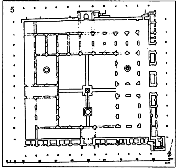
لوحة مجمعة 85: مخططات مساجد أفريقية القرن الثاني عشر: 1، 2: شمال، 3: الكتبية بمراكش، 4: المسجد السابق والمسجد الذي سبق، زال من الوجود اليوم؛ 5: من قصبة مراكش، 6: مسجد حسان بالرباط.
