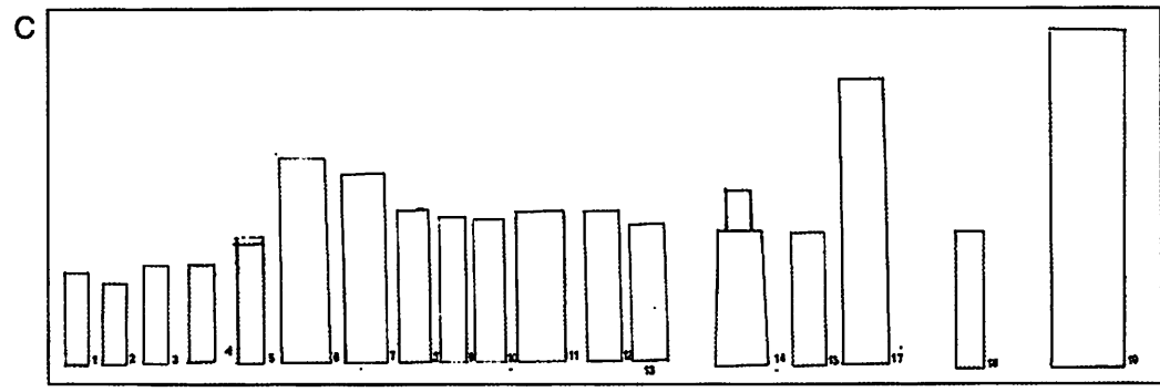
لوحة مجمعة 44: المنارات الإسبانية الإسلامية والمغربية. الارتفاعات.
